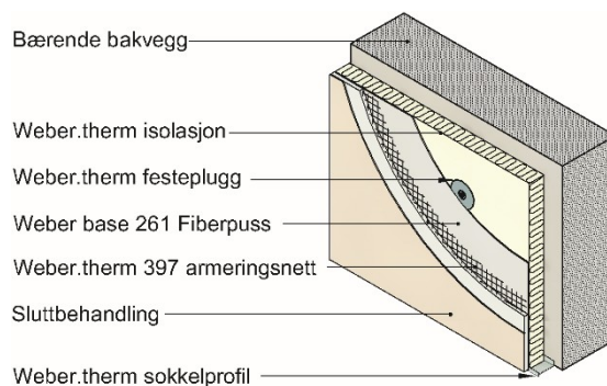
Fig. 1 Oppbygging av weber fasadesystemer
