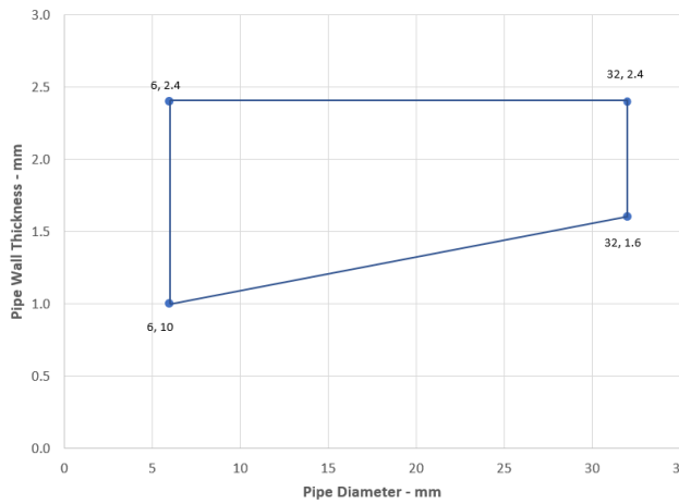
PVC-U Pipes EI 90 - U/C
