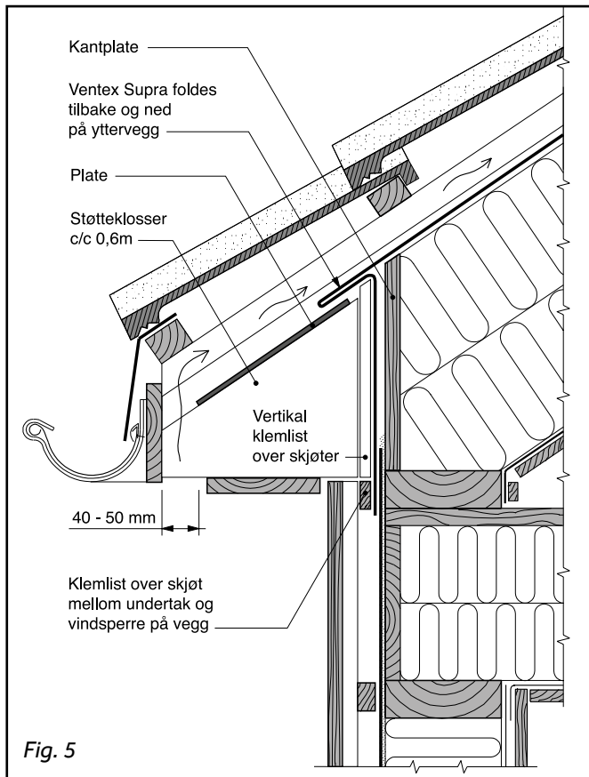
Fig. 5 Eksempel på overgang tak/yttervegg. Alternativ med avkuttete sperrer, der Ventex Supra føres sammenhengende over kontinuerlig kantplate eller kantbord og klemmes i omleggene med vindsperre på vegg.
