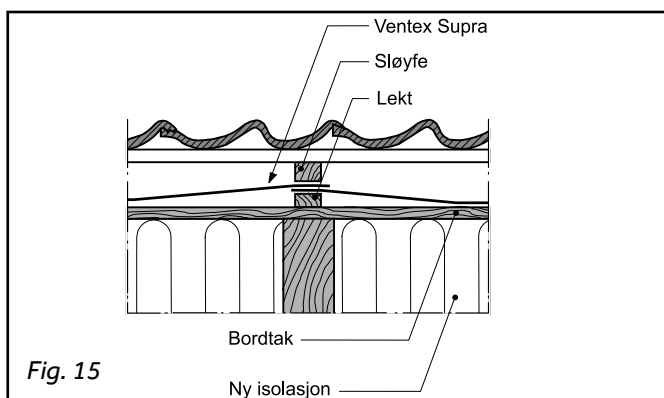
Fig. 15 Ventex Supra diffusionsåpent undertak montert på bordtak som er blitt fullisolert på undersiden. Hvis Ventex Supra monteres på gammelt bordtak, må diffusjonstett takbelegg fjernes. For å få tette omleggskjøter må det brukes lekter oppå bordtaket som skjøtene klemmes mot med sløyfene. Dette gir også fall bort fra skjøtene. Ved filt i sideomlegg skal Ventex Supra brettes tilbake, slik at filten ikke ligger eksponert.
