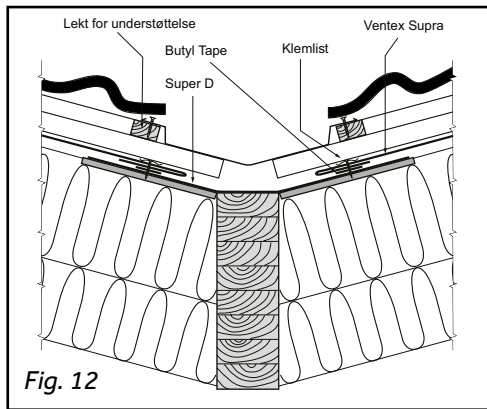
Fig. 12 Eksempel på utførelse av vinkelrenne med bygningsplate og membran av Icopal TopSafe eller Icopal Super D. Membranen kan erstattes med underbeslag. Det er viktig at undertaket holdes luft- og vannrett i vinkelrennen. Ventex Supra brettes tilbake, slik at filten ikke ligger eksponert. Omleggene kan event. suppleres med tette-masse.
