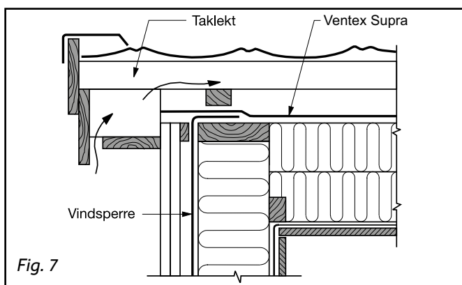
Fig. 7 Ventex Supra avsluttes ved gavlvegg slik at det blir en luftåpning under gavlutstikket. Det sikrer en effektiv krysslufing av taket. Ved filt i sideomlegg skal Ventex Supra brettes tilbake, slik at filteren ikke ligger eksponert.
