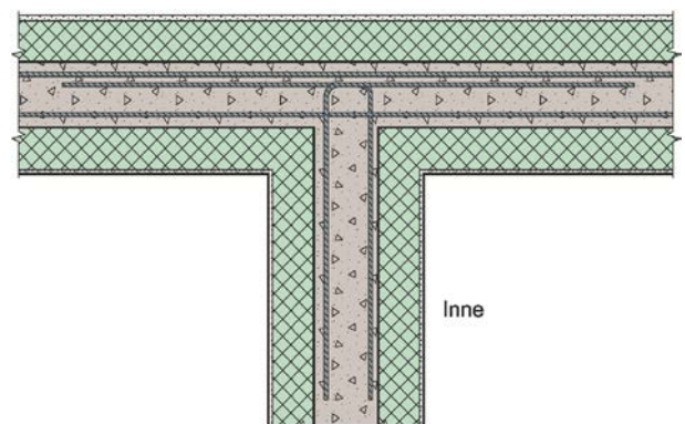
Fig. 12 Armering ved støttevegg for yttervegg mot terreng
