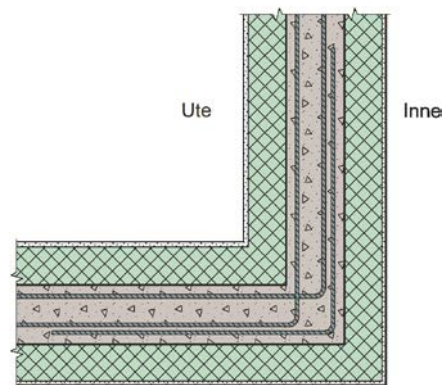
Fig. 10 Prinsipp for armering av innvendig hjørne
