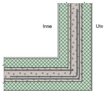
Fig. 11 Armering i utvendig hjørne for yttervegg mot terreng
