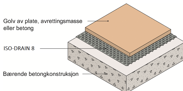
Fig. 2 Golvkonstruksjon med ISO-DRAIN 8 fuktsperre på betongdekke.
