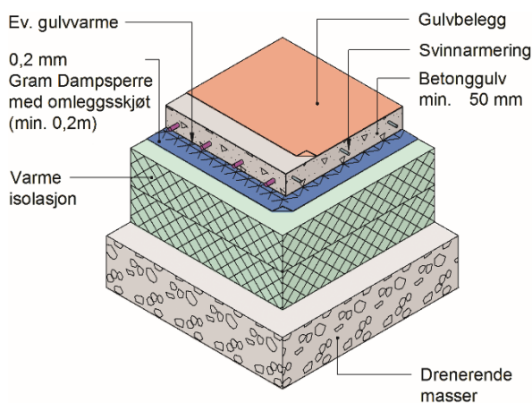
Fig 3 Gram Dampspærre og Gram Dampspærre av Fornybart Råstoff montert i betonggulv på grunnen
