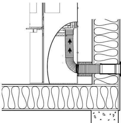
Durch Mauer
